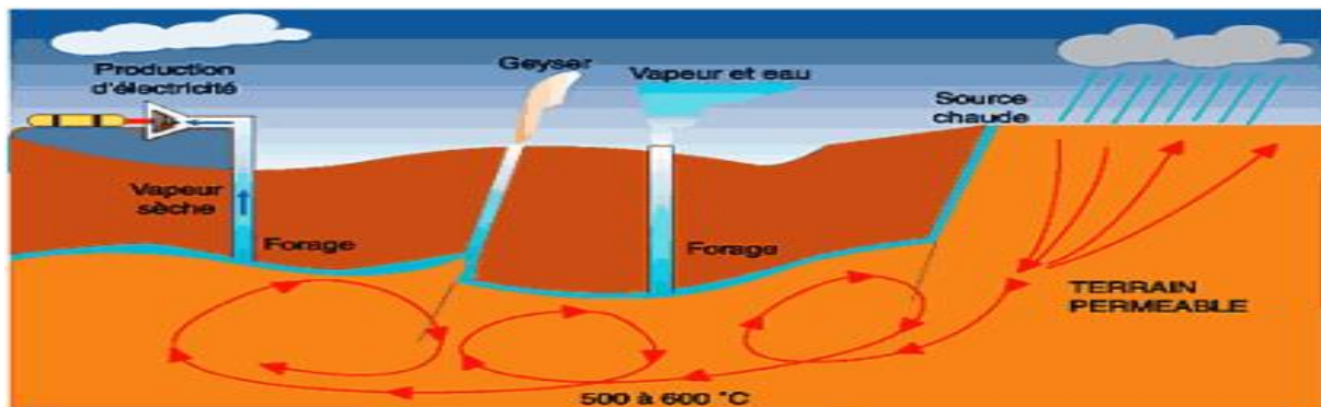
Figure 1 : Principe l'exploitation énergie géothermique
